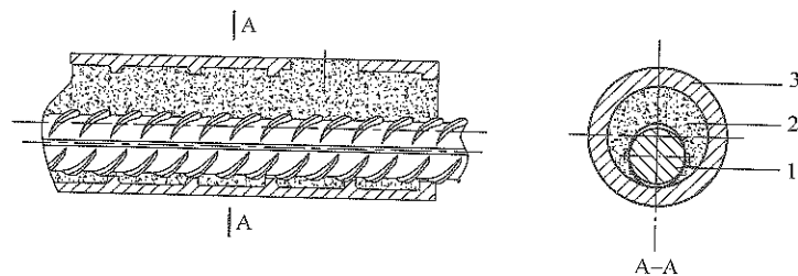
图1 偏置单向拉伸接头的钢筋偏置示意图
